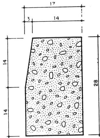
TIPO III 17 x 28 cm. PARA DELIMITACION DE ACERAS CON CALZADAS
